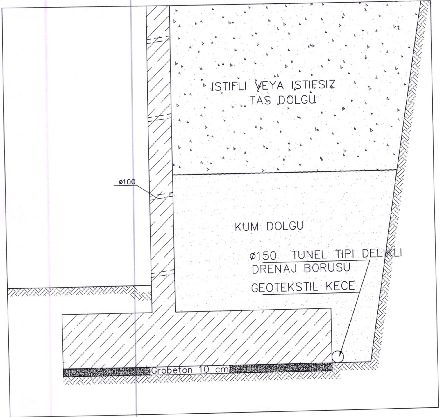
DRENAJ DETAYI
